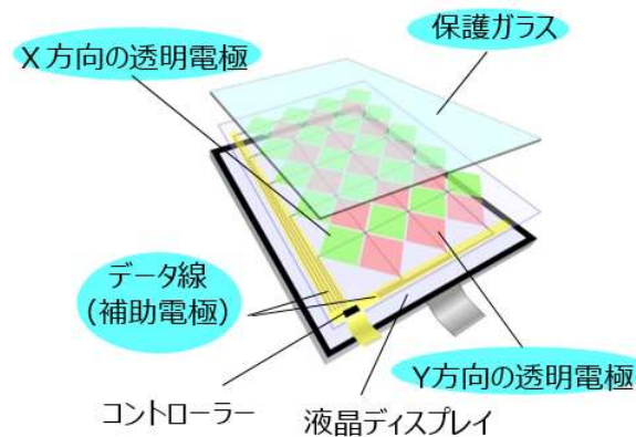
タッチパネルの構造
