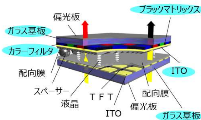
液晶ディスプレイの構造
